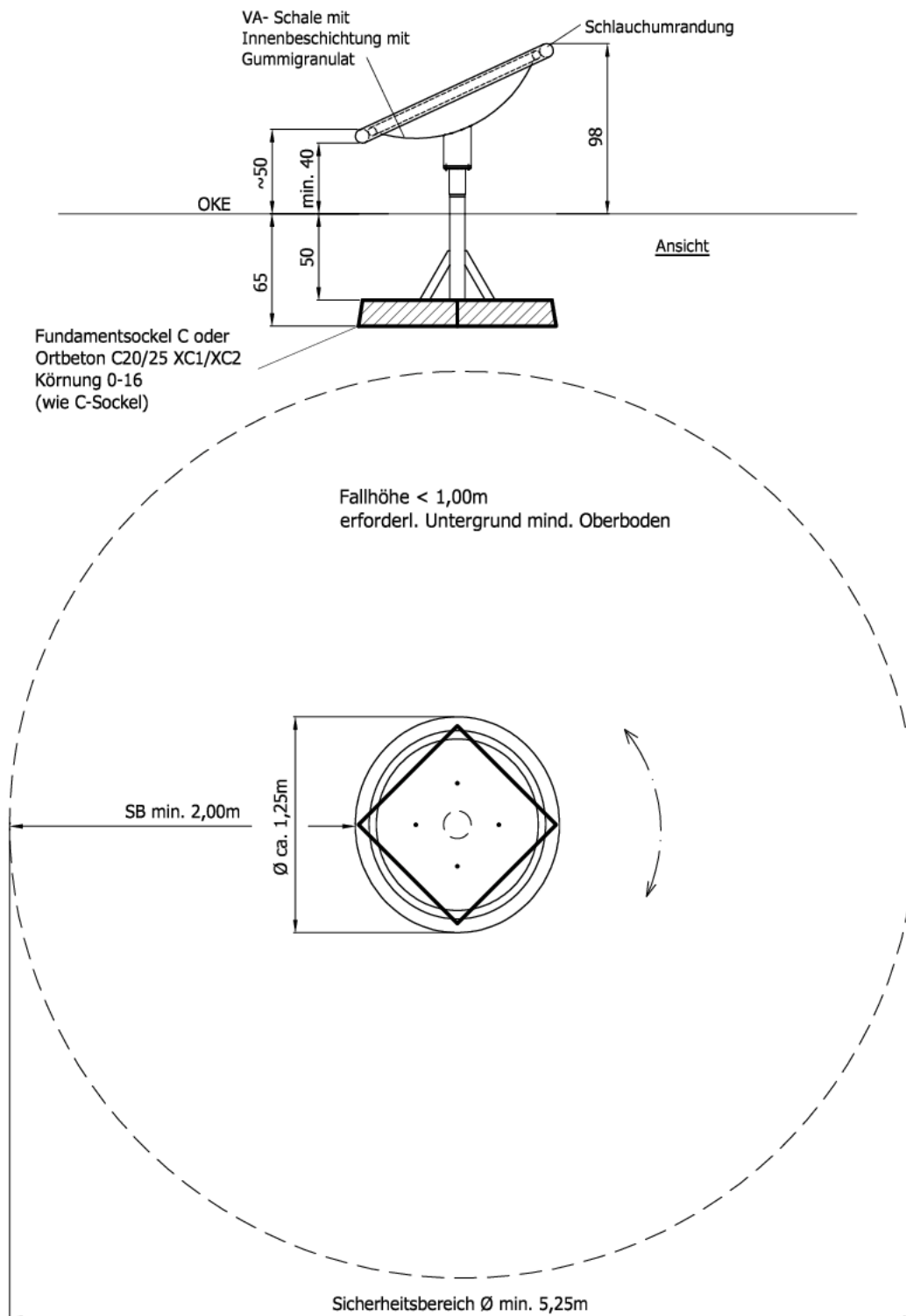
Fundamentsockel C Art-Nr.: 154003CS
