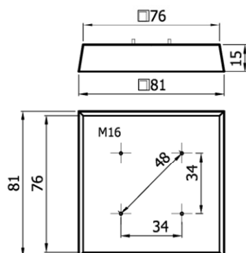
Fundamentsockel C Art-Nr.: 154003CS
